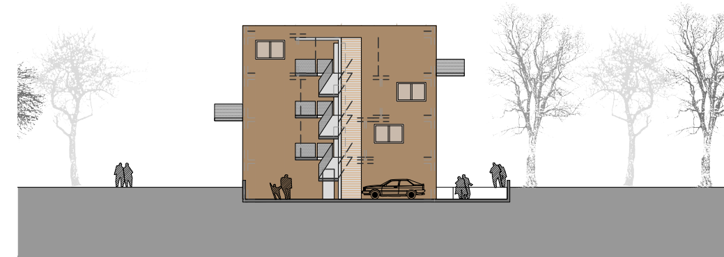
SCHNITT 2
