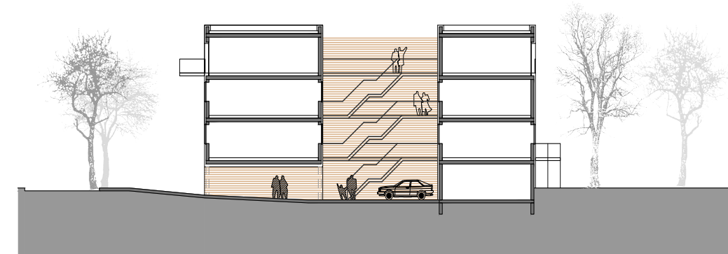
SCHNITT 1
