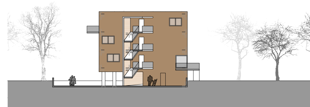
SCHNITT 3
